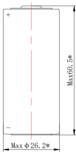
Dimensions in mm (GB1804-m)
