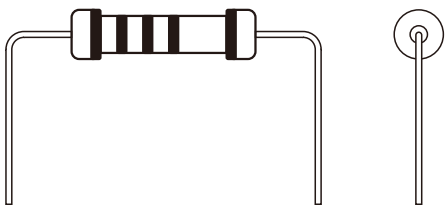
散装卧式MB形 Bulk horizontal MB type
