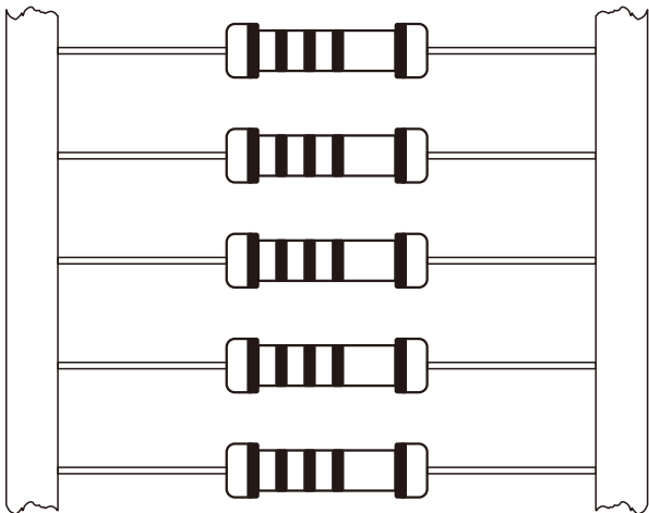
编带 盒装A形 A Tape/Box
