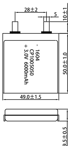
Dimensions in mm (GB1804-m)
