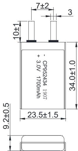
Dimensions in mm (GB1804-m)
