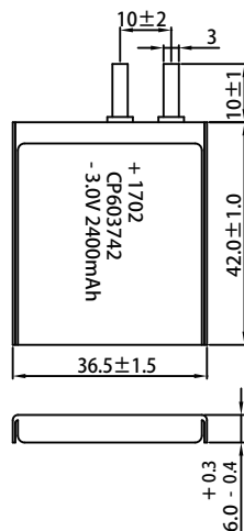
Dimensions in mm (GB1804-m)
