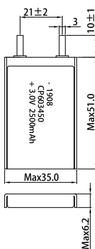
Dimensions in mm (GB1804-m)
