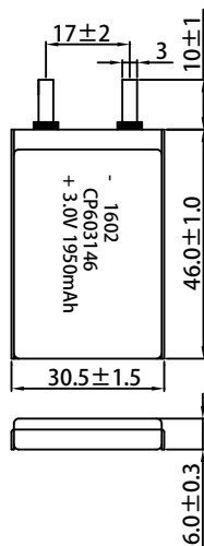
Dimensions in mm (GB1804-m)
