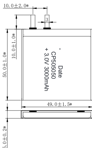
Dimensions in mm (GB1804-m)
