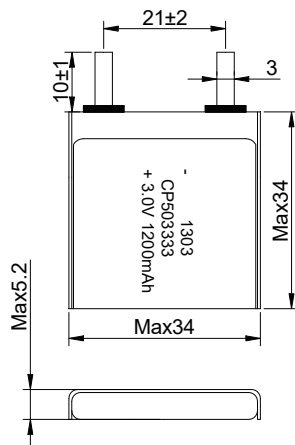
Dimensions in mm (GB1804-m)
