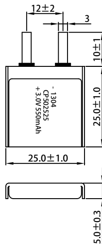
Dimensions in mm (GB1804-m)
