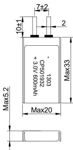
Dimensions in mm (GB1804-m)
