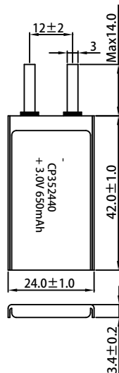
Dimensions in mm (GB1804-m)
