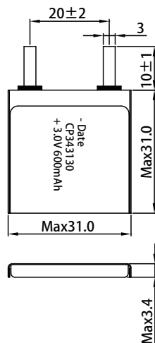
Dimensions in mm (GB1804-m)
