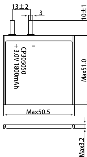
Dimensions in mm (GB1804-m)
