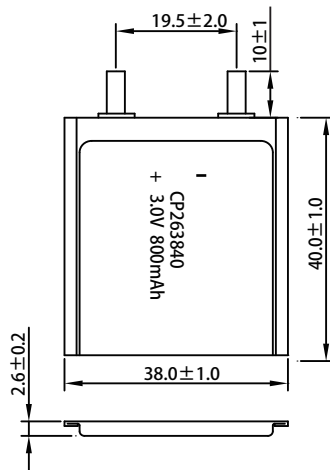
Dimensions in mm (GB1804-m)
