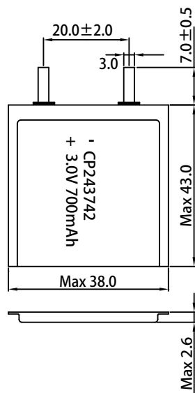
Dimensions in mm (GB1804-m)
