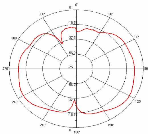
2.45 GHz H-Plane vertical
