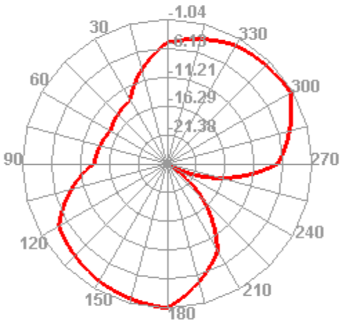
960.000MHz E1
