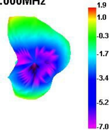
1710.000MHz
