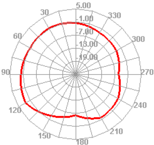
1710.000MHz H
