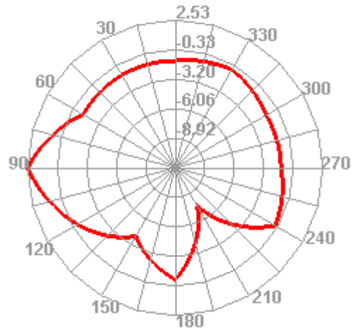
2300.000MHz E2
