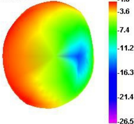
960.000MHz
