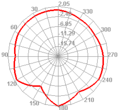
820.000MHz E2
