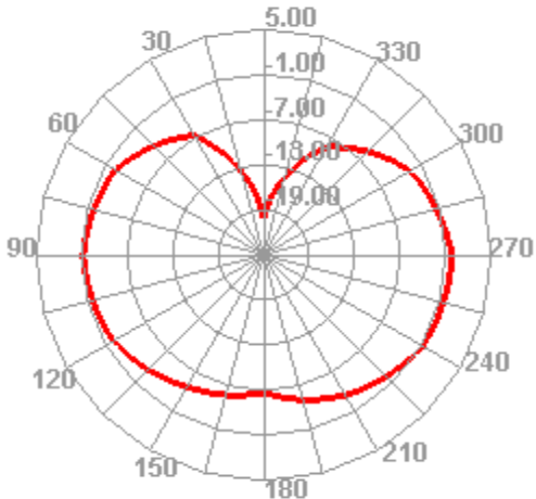
820.000MHz H
