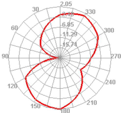
820.000MHz E1
