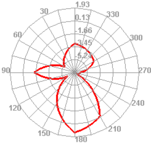
1710.000MHz E1
