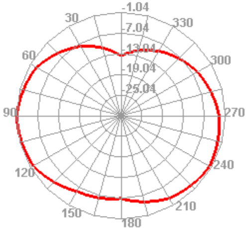
960.000MHz H
