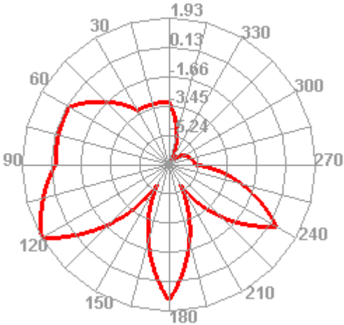
1710.000MHz E2
