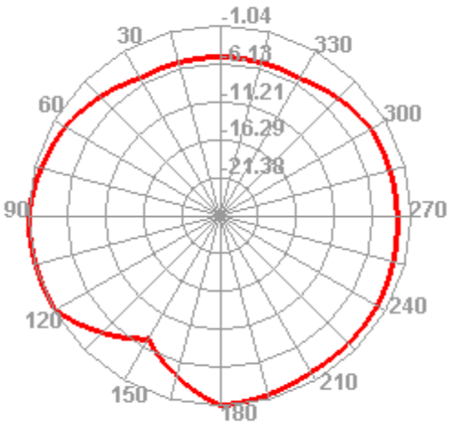
960.000MHz E2
