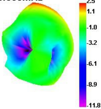
2300.000MHz
