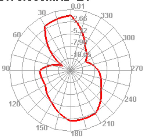
2170.000MHz E1
