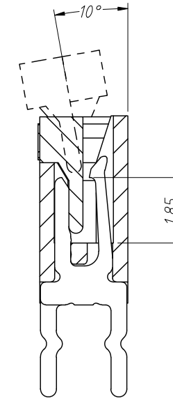
SECTION A-A
