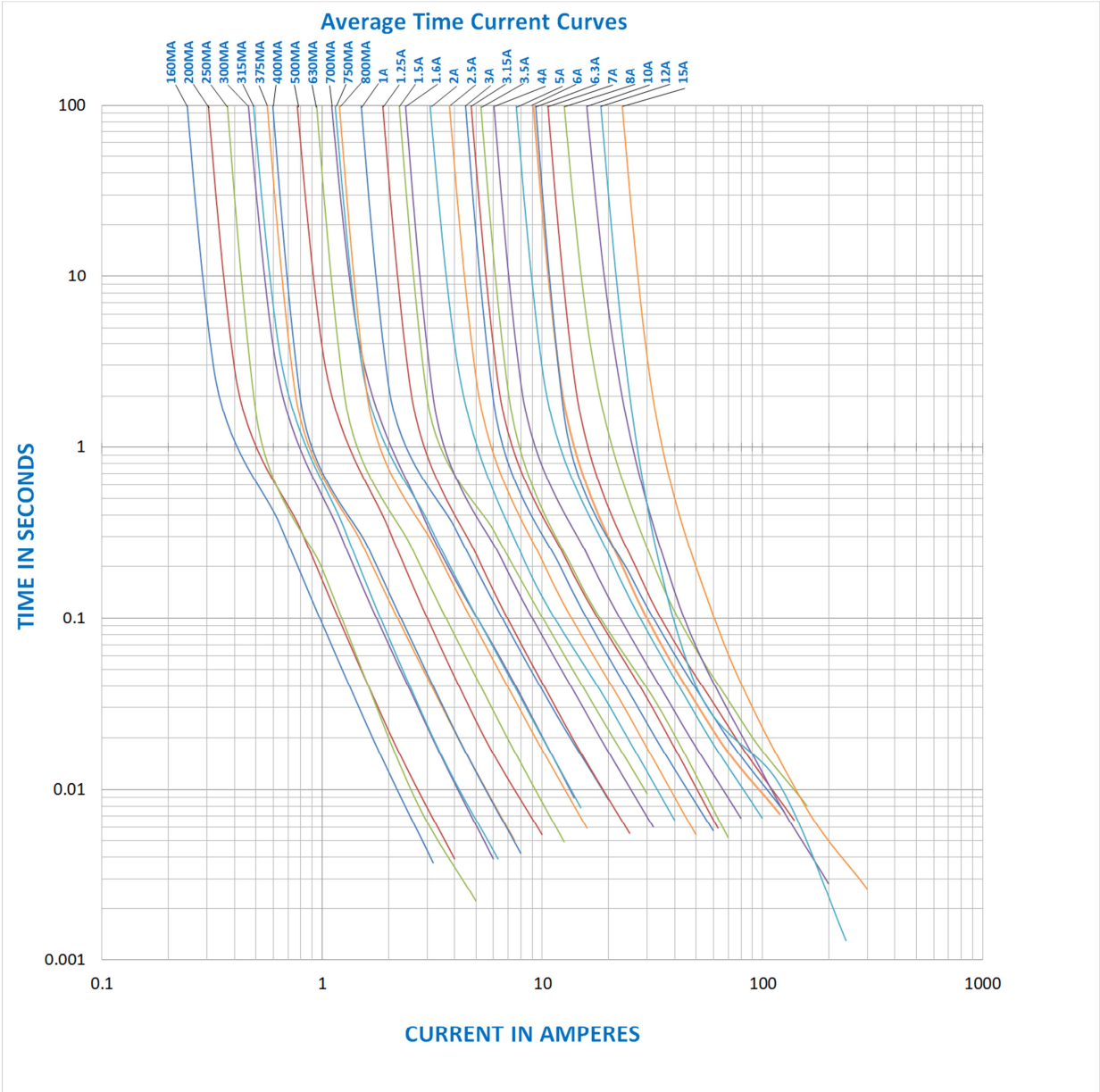
7.4 平均时间电流曲线图 / Average Time Current Curves
