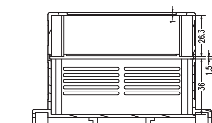
剖面 A-A
