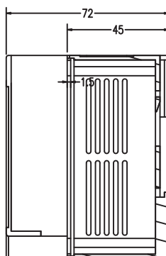
剖面 B-B
